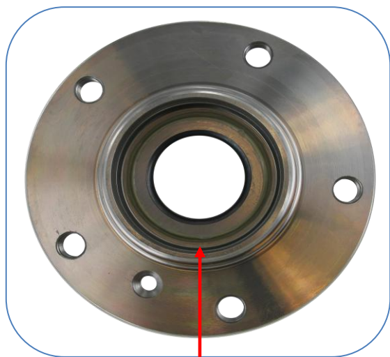
A/M kialakítás- külső oldali tömítéssel
