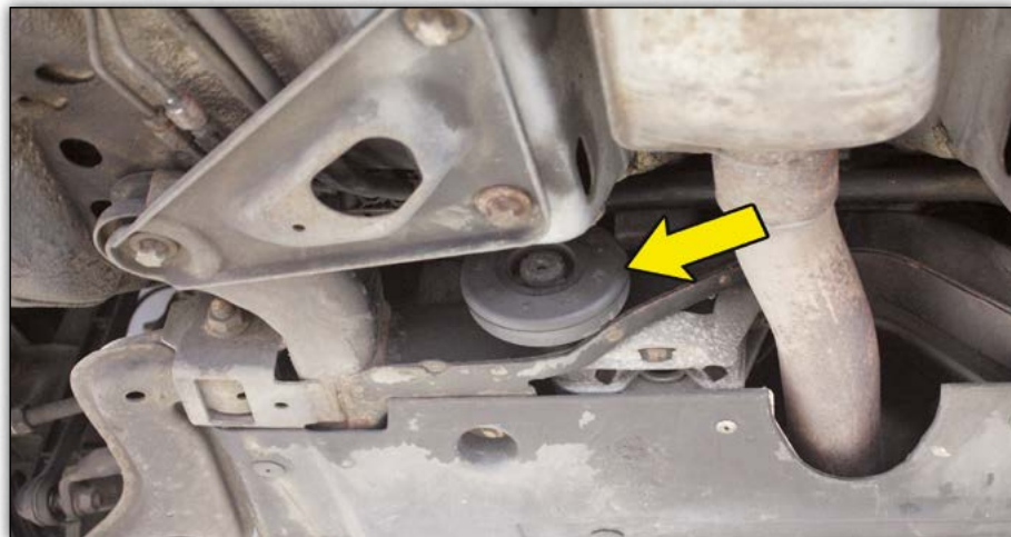
1. ábra: Lengéscsillapító beszerelt állapotban
