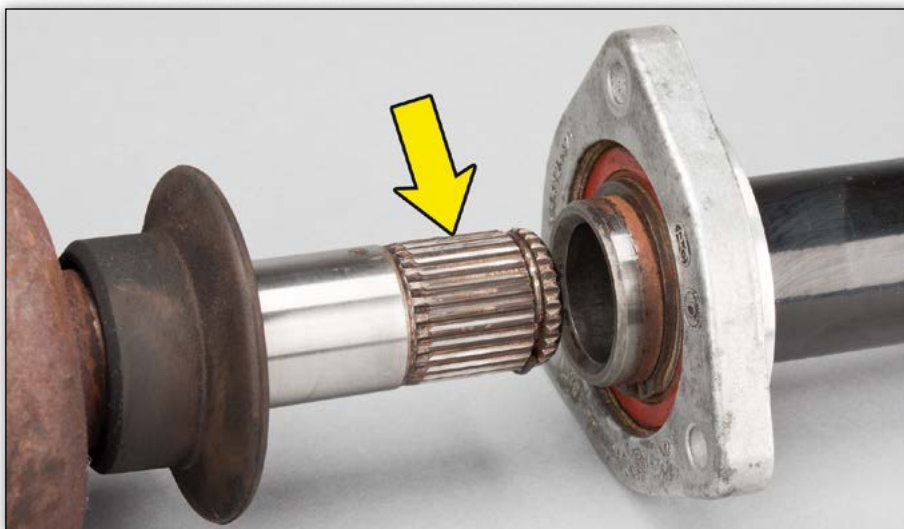
1. ábra: Kenőanyagbeviteli hely a meghajtótengely csatlakozásán
