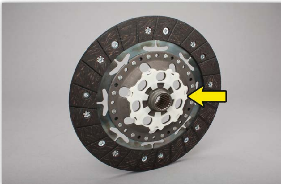
1. ábra: LuK kuplungtárcsa műanyag gyűrűvel
