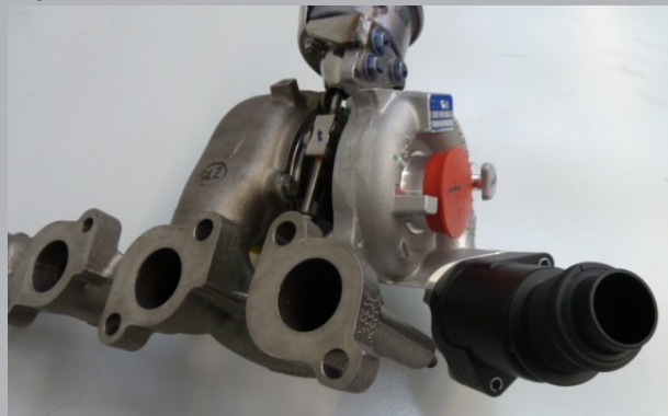
Turbó hangcsillapítással
